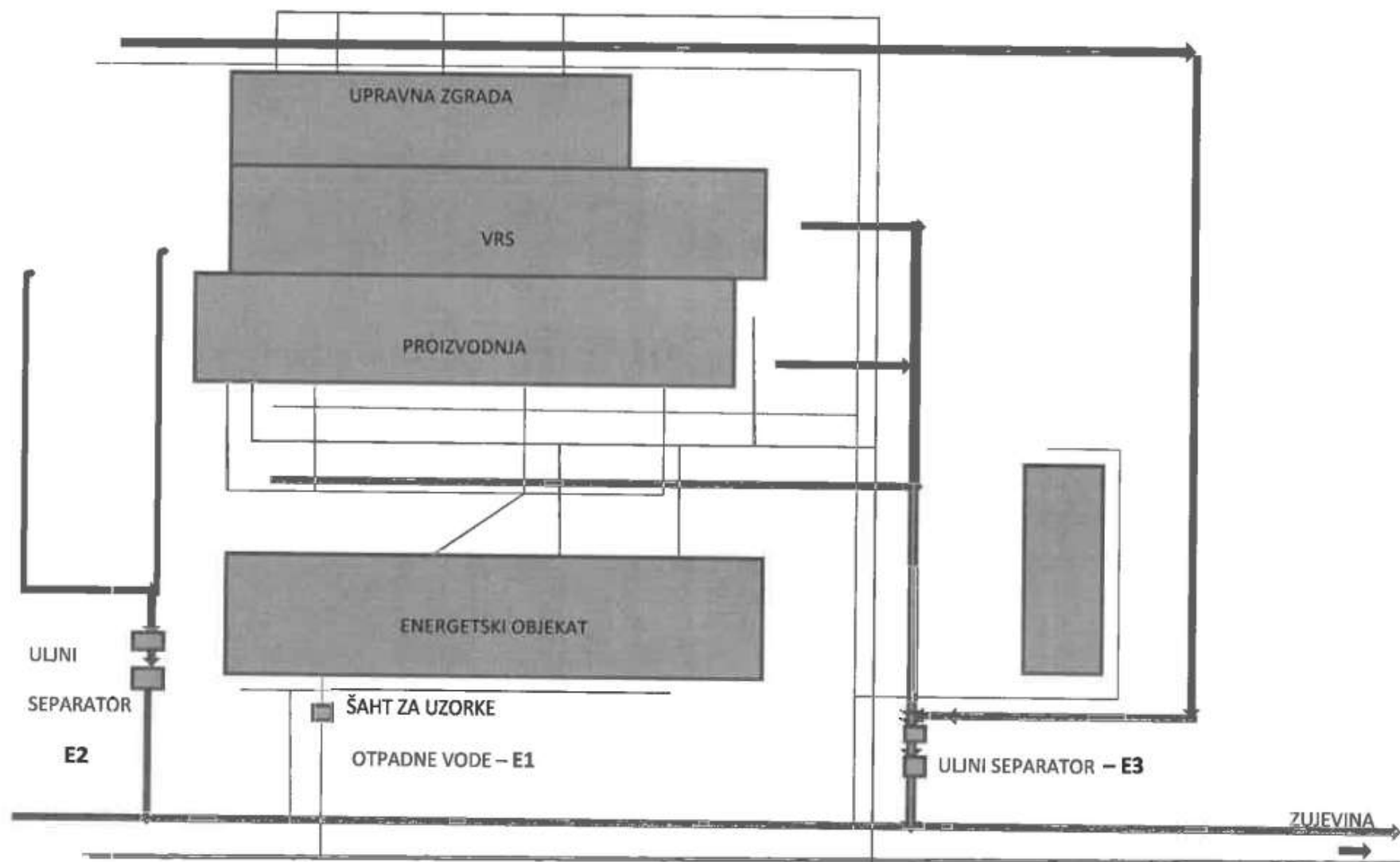
ATLANTIC ARGETA - UPROŠĆENA ŠEMA OTPADNIH VODA
