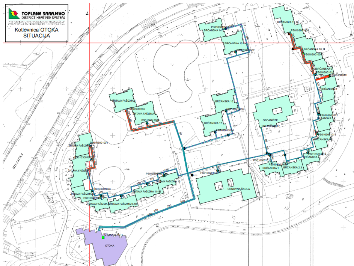
Slika 3. Situacioni prikaz kotlovnice sa postojećom distributivnom mrežom
