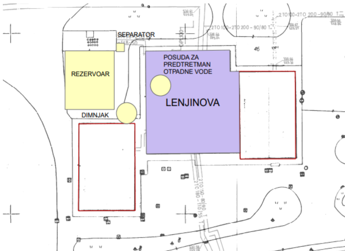
Slika 4. Dispozicija objekata u kotlovnici
