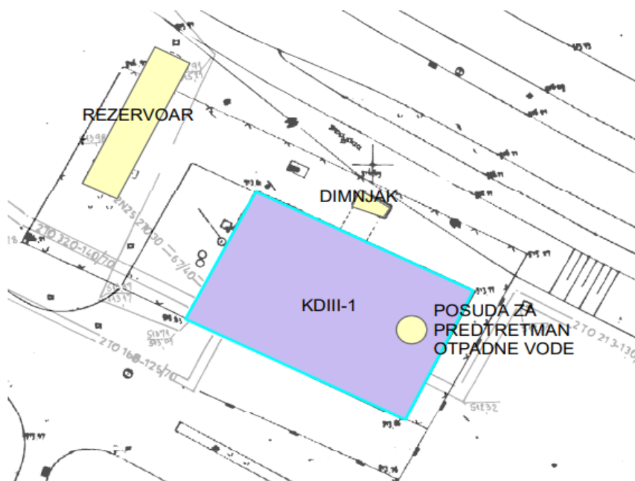
Slika 4. Dispozicija objekata u kotlovnici
