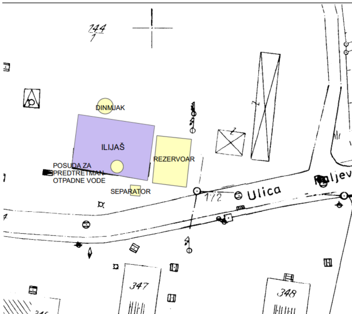
Slika 4. Dispozicija objekata u kotlovnici
