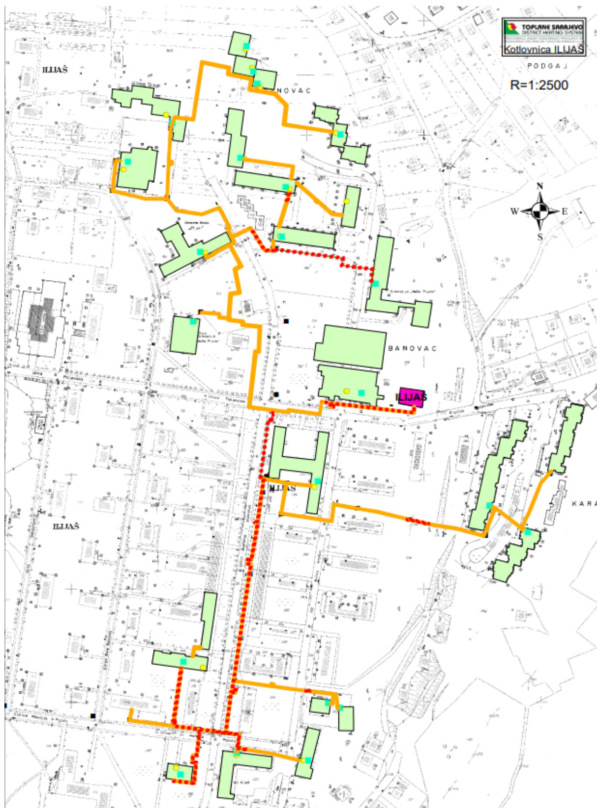
Slika 3. Situacioni prikaz kotlovnice sa postojećom distributivnom mrežom
