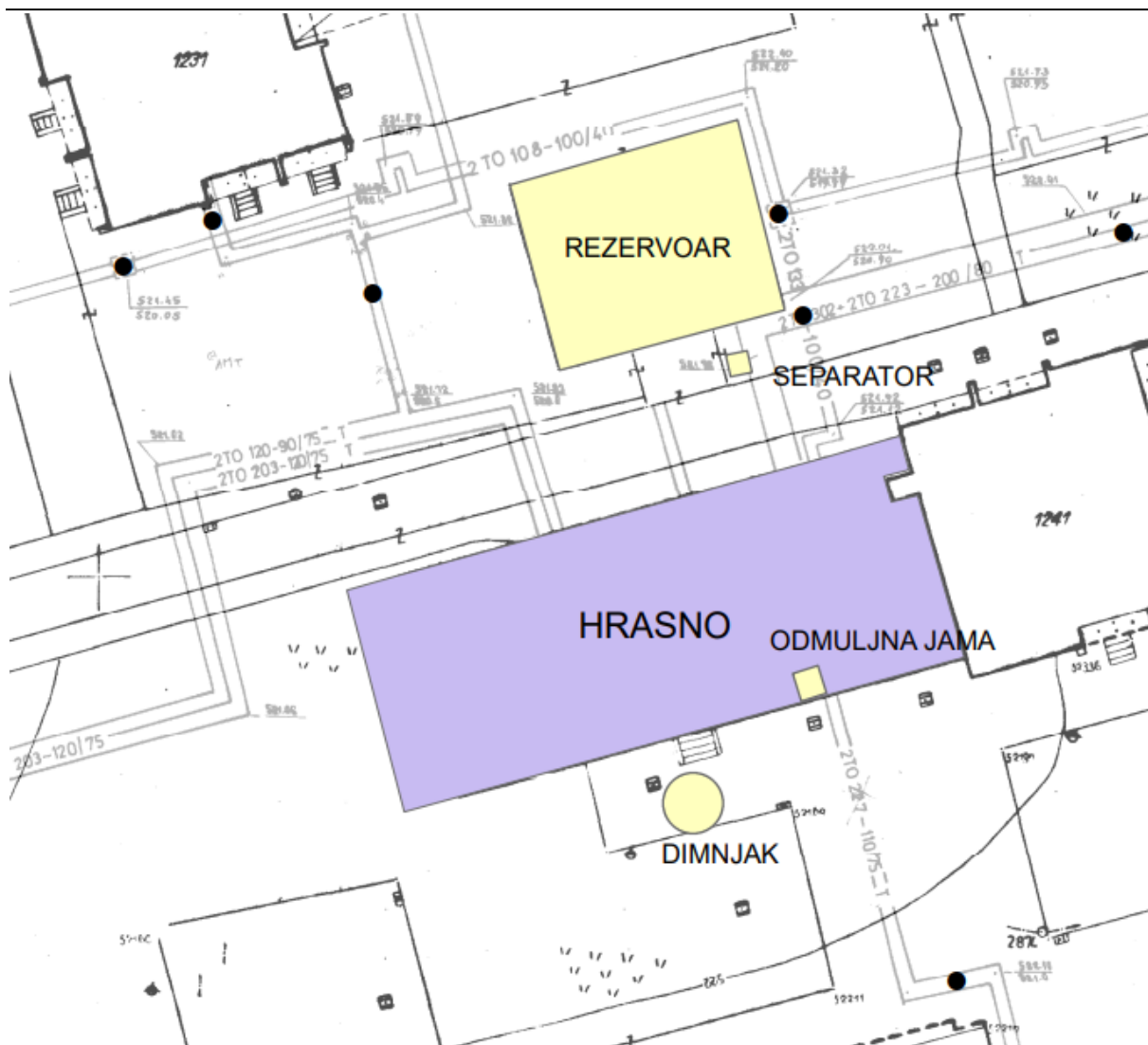
Slika 4. Dispozicija objekata u kotlovnici
