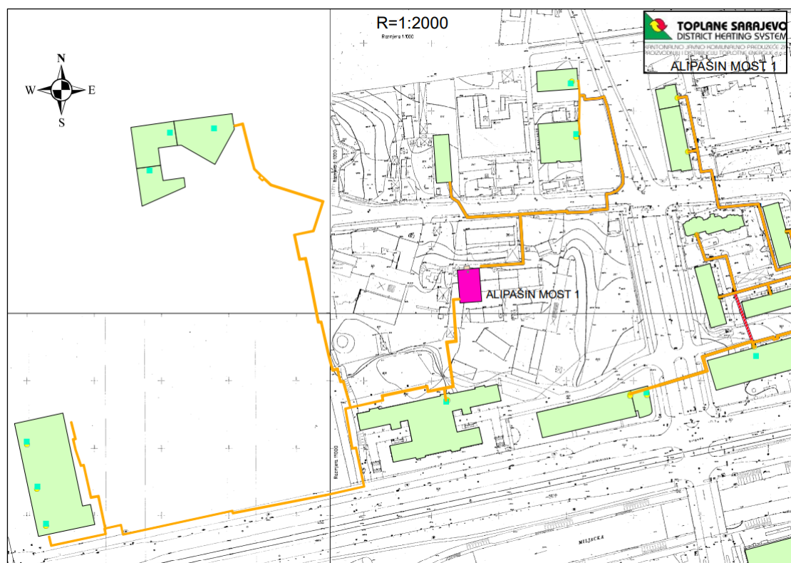
Slika 3. Situacioni prikaz kotlovnice sa postojećom distributivnom mrežom
