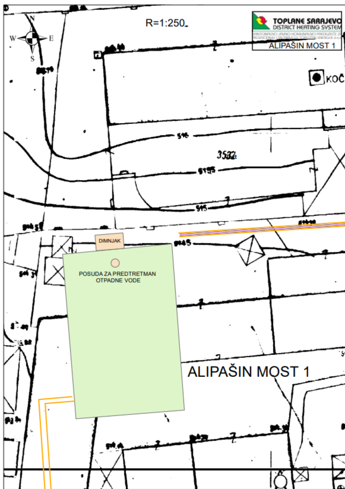
Slika 4. Dispozicija objekata u kotlovnici
