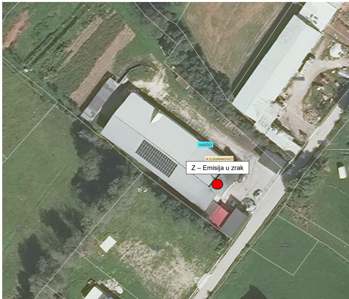
Tlocrt pogona/postrojenja sa mjestima emisija
