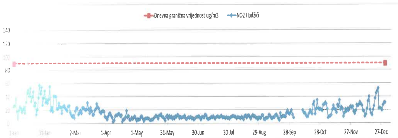
Dijagram 9. Prosječne dnevne koncentracije NO 2 tokom 2022.
