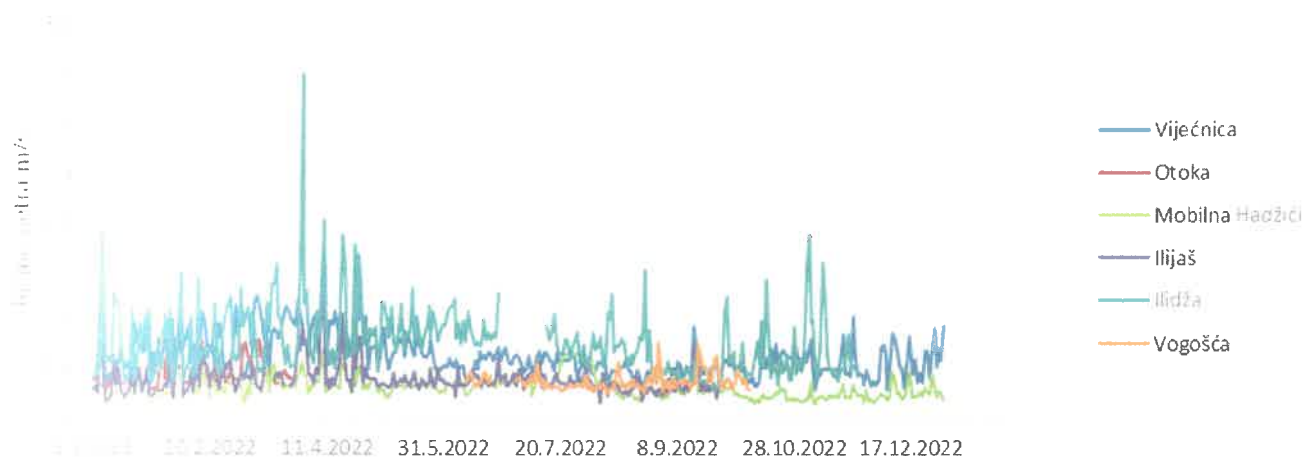
Dijagram 22. Prosječne dnevne brzine vjetra na stanicama tokom 2022.
