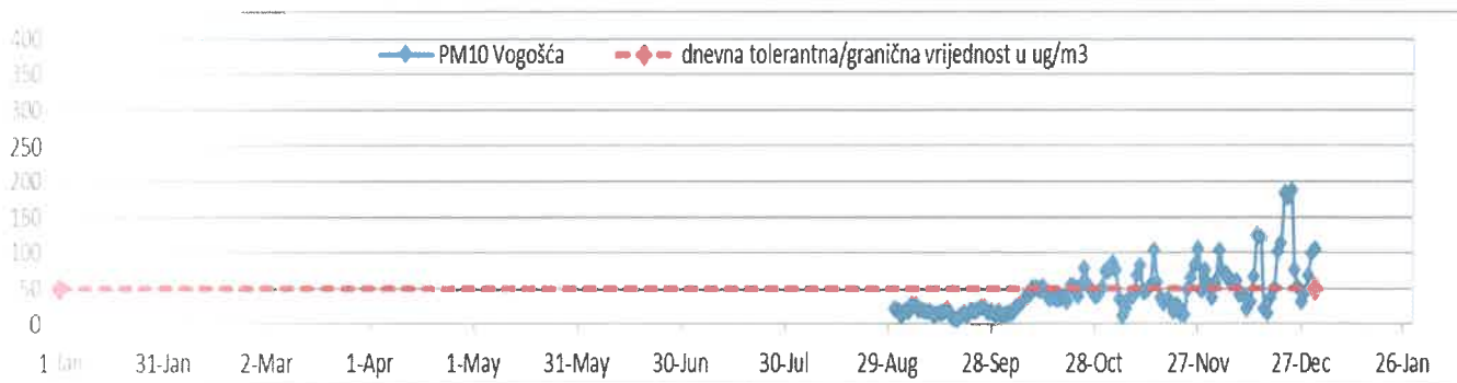
Dijagram 13. Prosječne dnevne koncentracije PM 10 tokom 2022.
