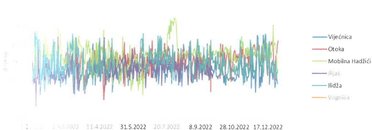
Dijagram 23. Prosječni dnevni smjerovi vjetra na stanicama tokom 2022.
