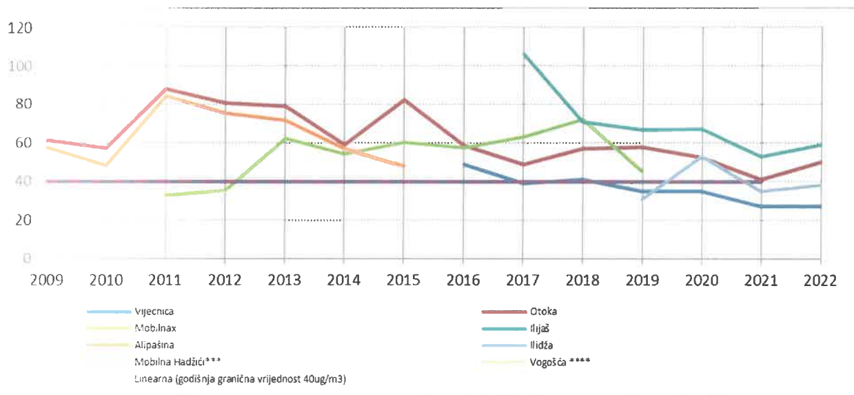
Dijagram 27. Prikaz kretanja koncentracije PM 10 tokom svih godina praćenja automatskim stanicama
