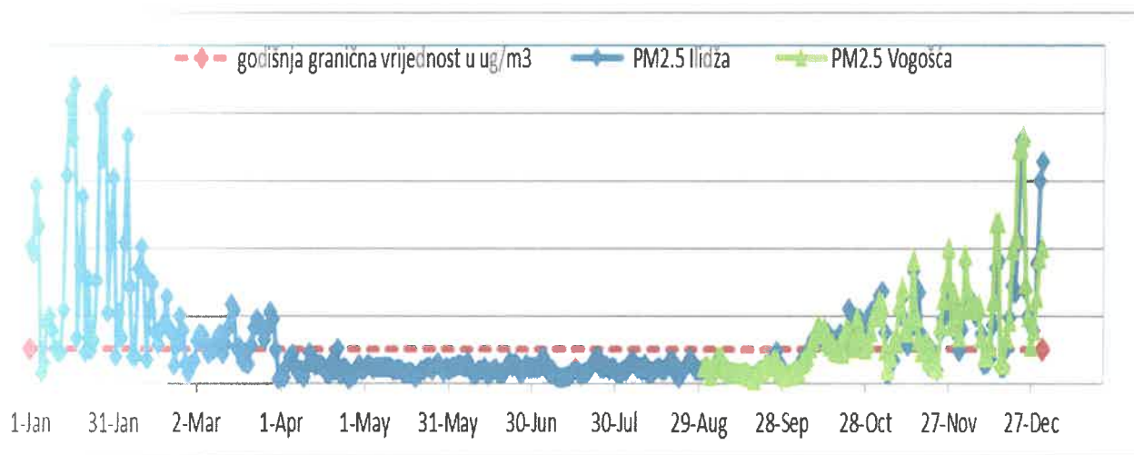
Dijagram 19. Prosječne dnevne koncentracije PM 2,5 tokom 2022. mjerene automatskim stanicama
