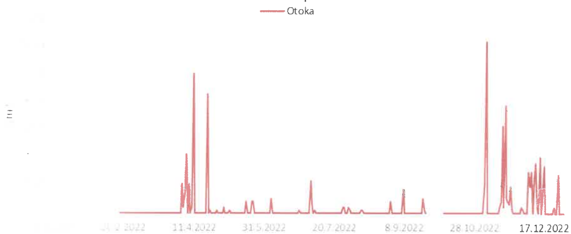
Dijagram 24. Prosječna količina padavina tokom 2022.
