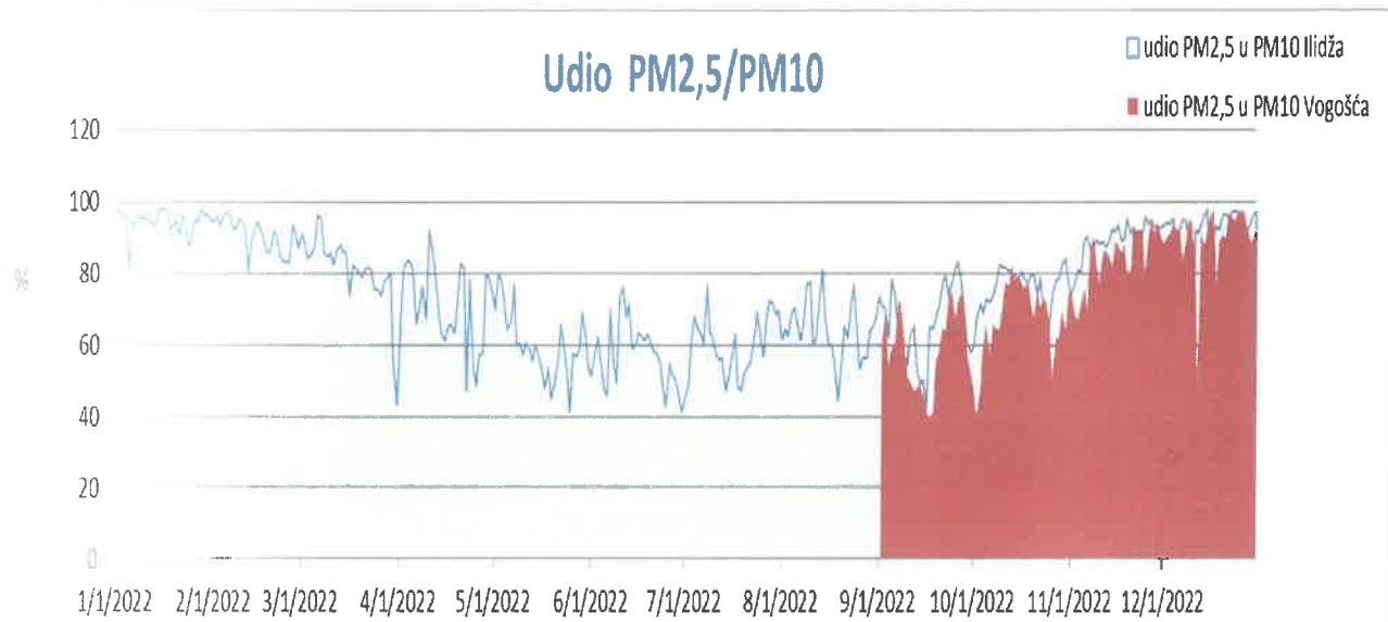
Dijagram 28. Udio PM_{2,5} u PM_{10} tokom 2022.
