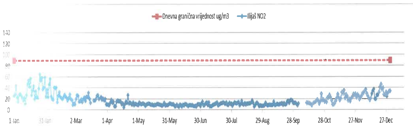
Dijagram 12. Prosječne dnevne koncentracije NO 2 tokom 2022.
