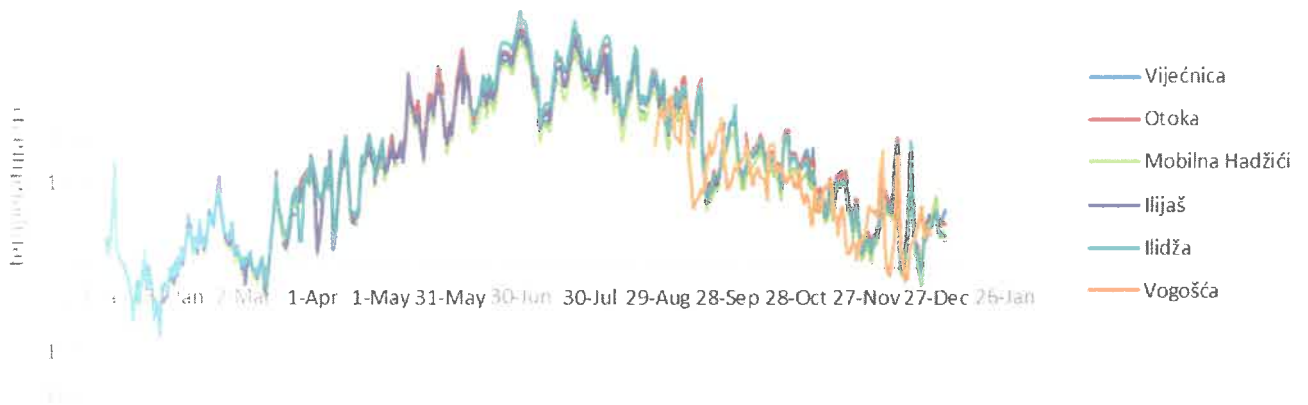
Dijagram 21. Prosječne dnevne temperature na stanicama tokom 2022.
