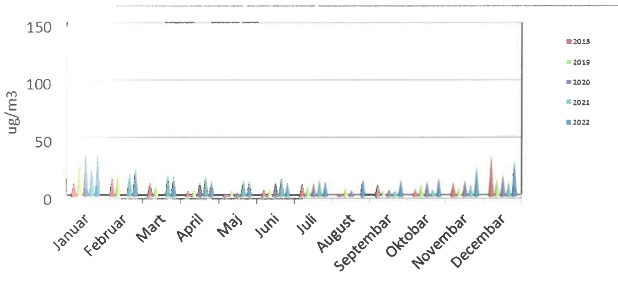
Dijagram 34. Prikaz kretanja koncentracije sumpor dioksida tokom posljednje pet godina praćenja automatskom stanicom prema mjesecima
