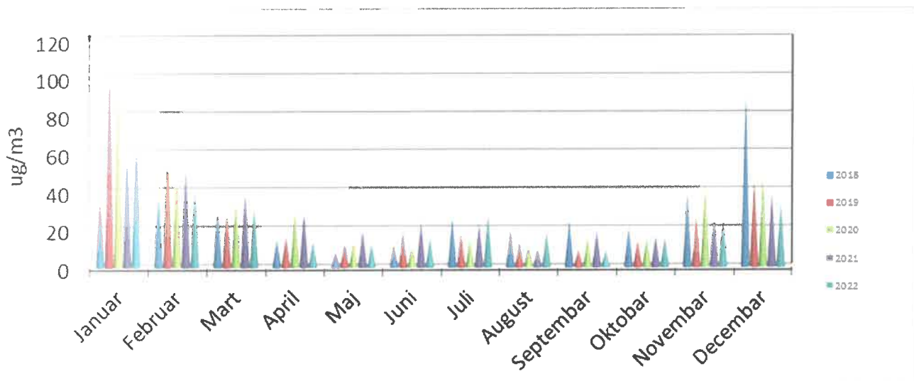
Dijagram 33. Prikaz kretanja koncentracije sumpor dioksida tokom posljednjih pet godina praćenja automatskom stanicom prema mjesecima
