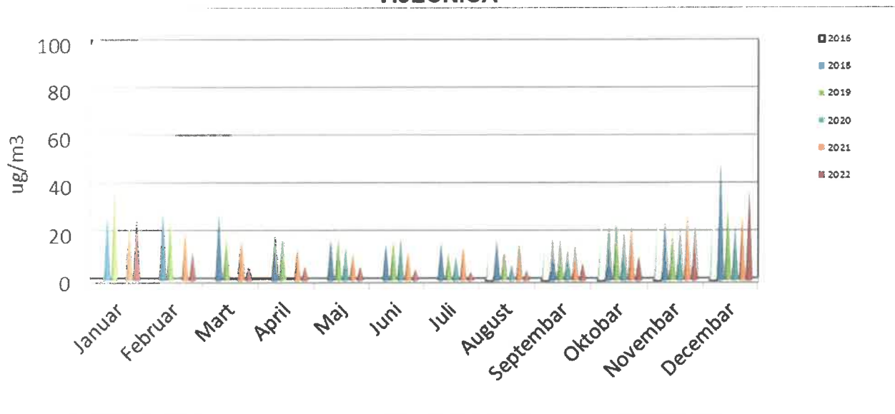
Dijagram 36. Prikaz kretanja koncentracije azot dioksida tokom posljednjih pet godina praćenja automatskom stanicom prema mjesecima
