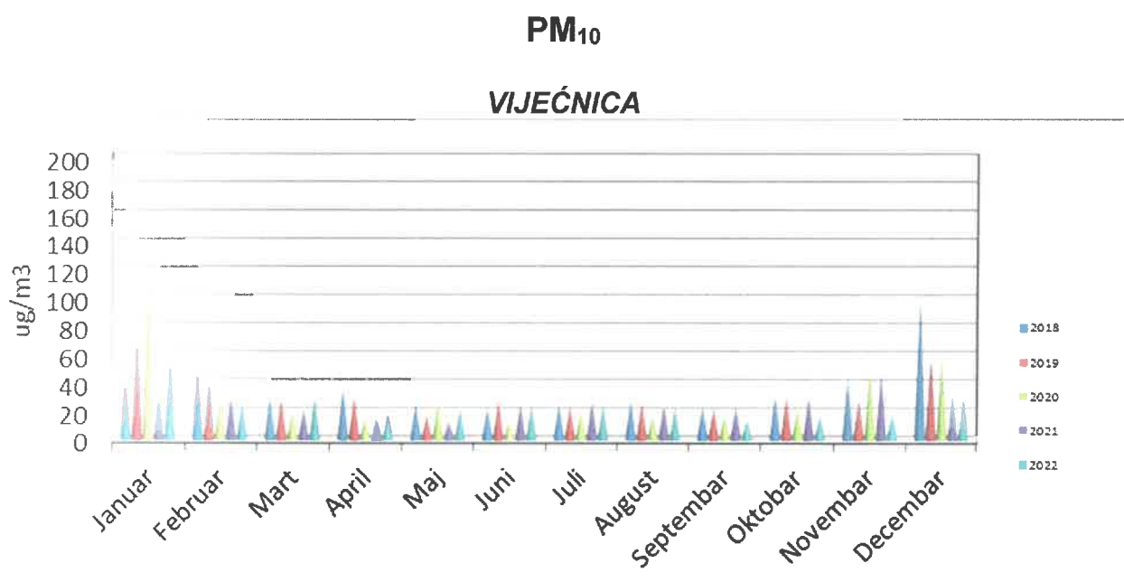
Dijagram 29. Prikaz kretanja koncentracije PM_{10} tokom posljednjih pet godine praćenja automatskom stanicom prema mjesecima
