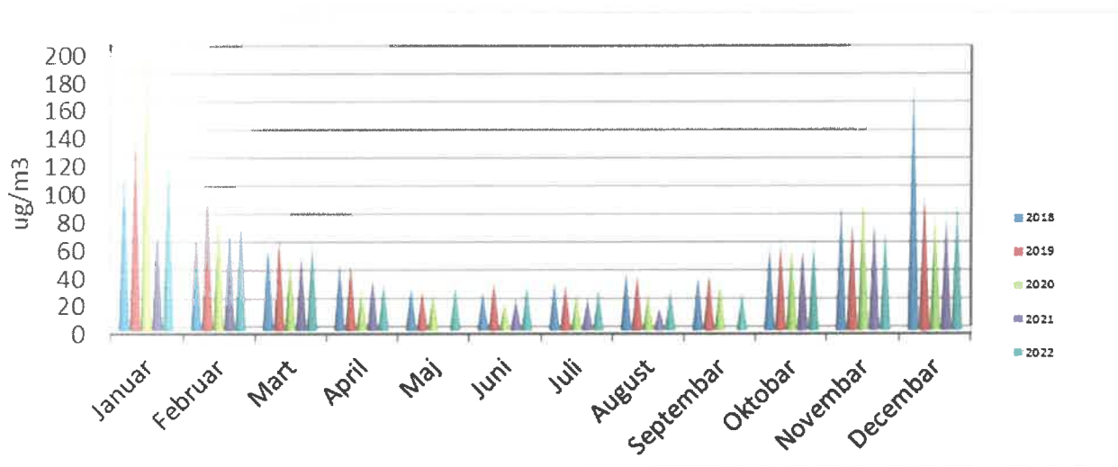
Dijagram 31. Prikaz kretanja koncentracije PM 10 tokom posljednjih pet godina praćenja automatskom stanicom prema mjesecima
